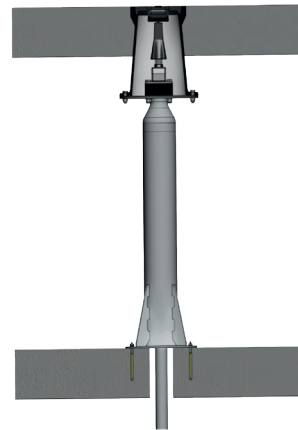
Unterflur-Antrieb Typ FSV
